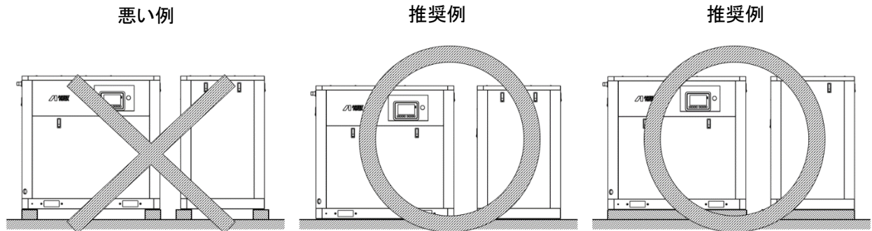
図4.3-1 設置方法例
