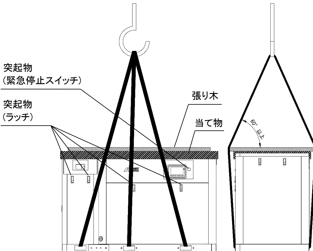
図4.2.2 クレーン等による運搬
